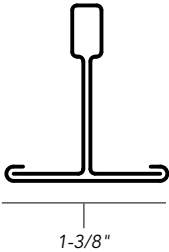
640/650 Drywall Grid
