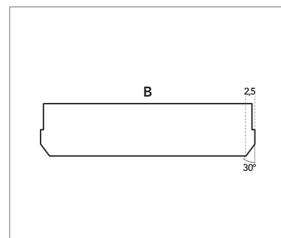
Systemet kan användas för direktmontering med kant B.
