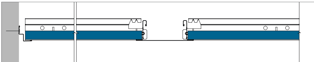
Wykończenie za pomocą kątownika przyściennego schodkowego W.
