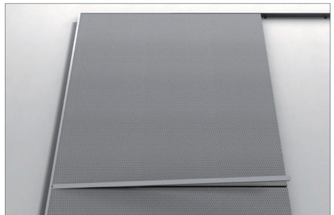
3.6 Bedek de horizontale voegen tussen de panelen door T24-profielen in de T-bevestigingssteunen te klikken. Schuif ze vervolgens voorzichtig onder de rand van het randprofiel. Deze horizontale T-stukken moet u afzagen op exact M-12 mm.
