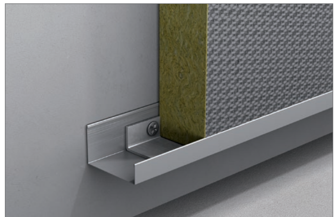
3.4 Gebruik indien nodig steunbeugels aan de binnenkant van de onderste J-randprofielen.
