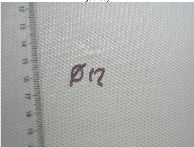
Constat de perforation partielle \varnothing 12 mm (énergie 3,75 joules)
