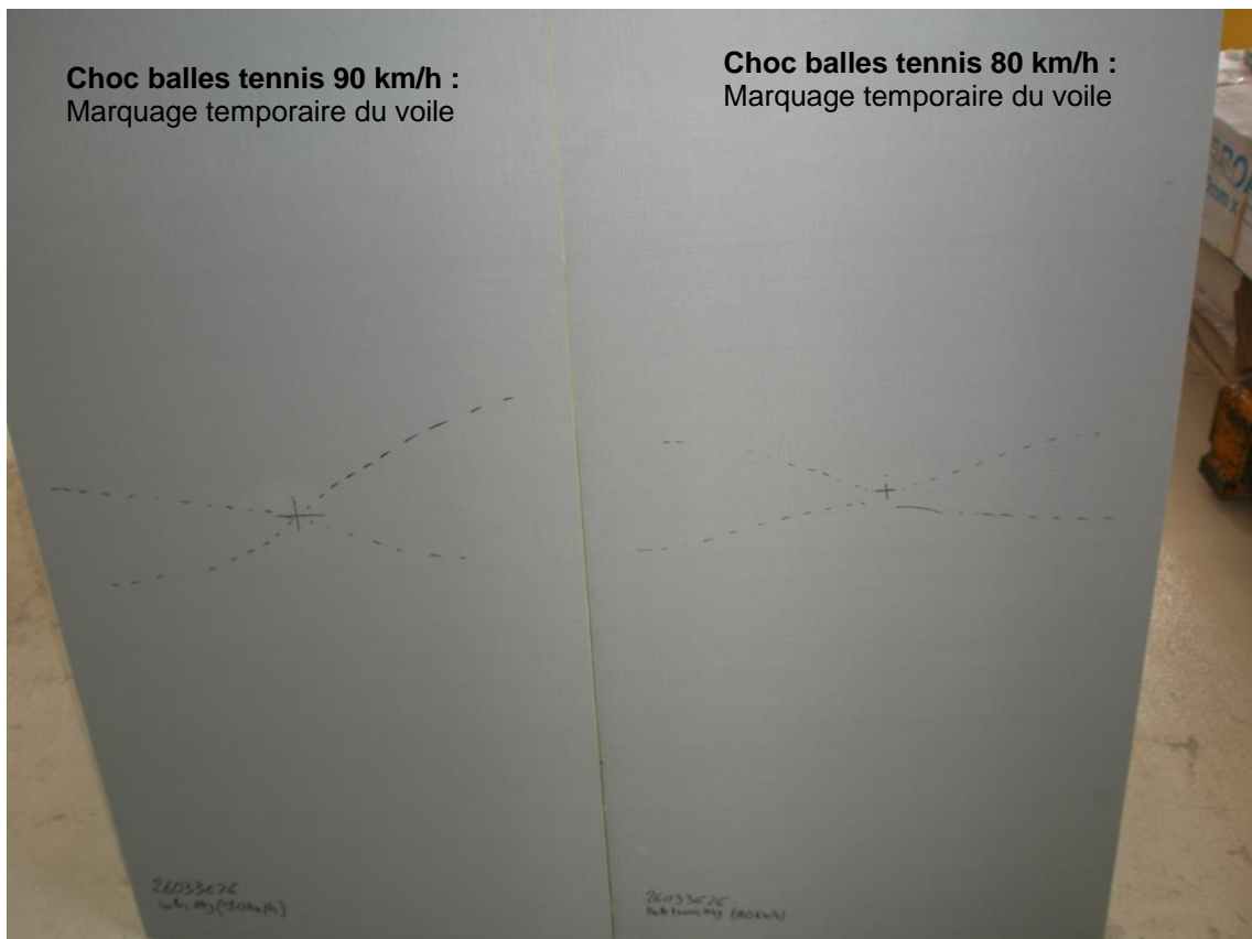
Photographie n° 16 : Essai de choc de balles de tennis lestées sur VertiQ 1200x600x40mm
