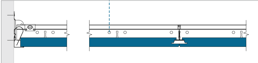
Finition périphérique avec cornière de rive. La pièce de raccord pour murs et chevêtres permet de positionner parfaitement la hauteur du porteur par rapport à la cornière.
