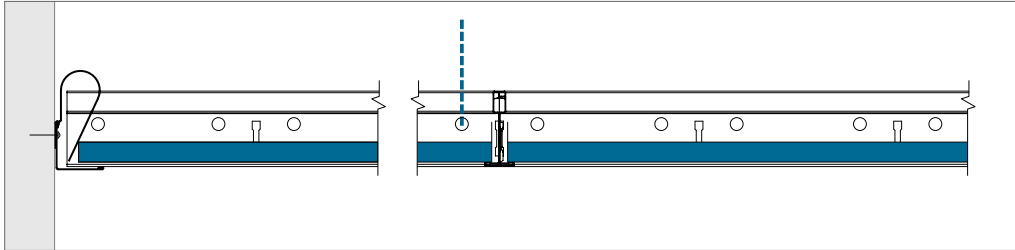
A-kant - kantafslutning med vinkelkantprofil. Kantfjeder kan anvendes efter behov.
