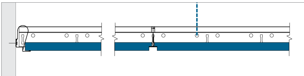
E-kant - kantafslutning med skyggenotsprofil. Kantfjeder kan anvendes efter behov
