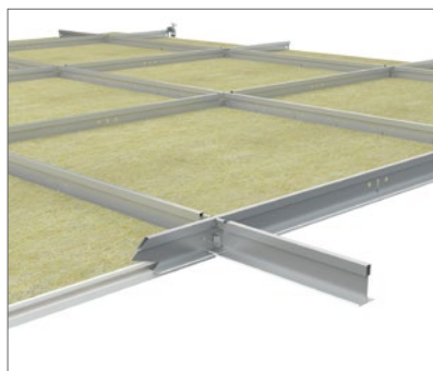
Trag- und Querschienen mit einer einheitlichen Höhe von 38 mm für eine hohe Stabilität und den einfachen Einbau von Serviceinstallationen. Das Klicksystem sorgt für einfache und schnelle Montage und Demontage.
