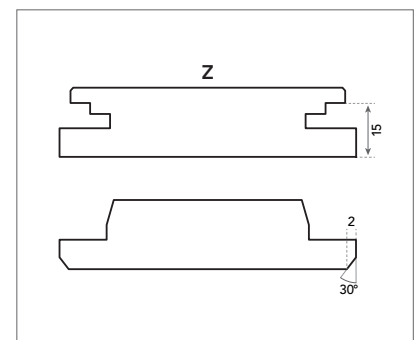
Z-Kante Detail: Die Z-Kante erzeugt im Deckenbild entlang der tragenden Plattenkante eine geradlinige Schattenfuge, die nichttragende Kante verdeckt die Unterkonstruktion.
