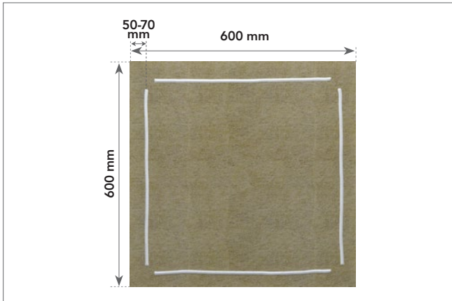
Klebeschema 1
