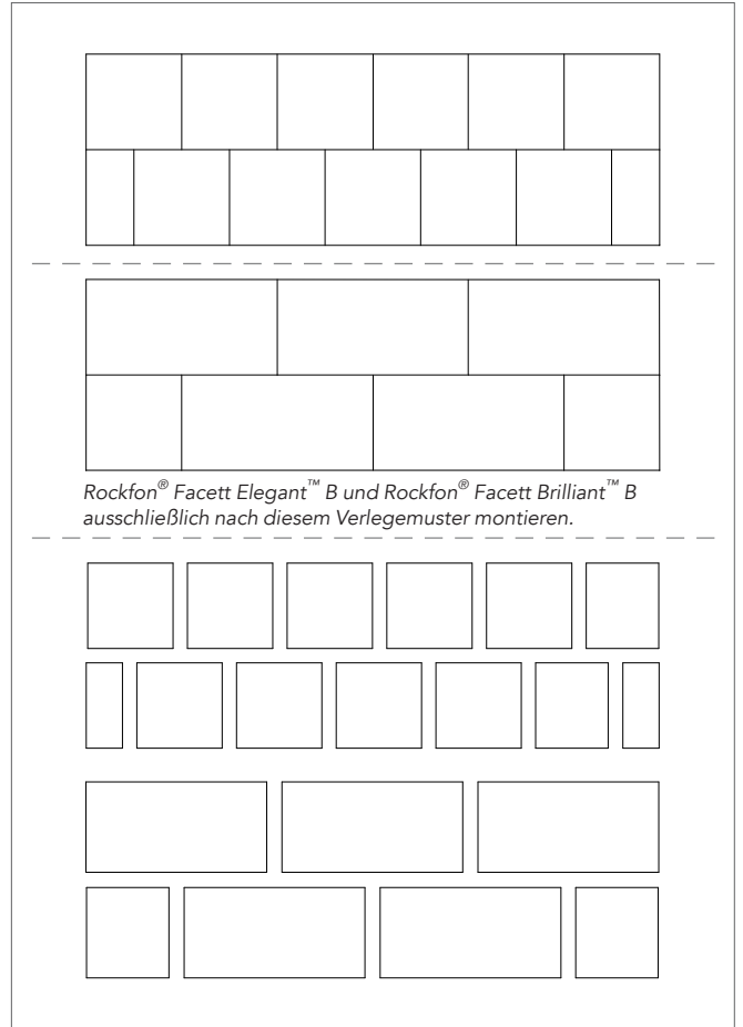
Im Verband.
