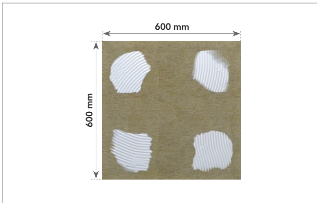
Klebeschema 2
