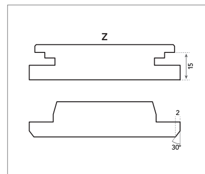
Details kantafwerking Z creëert een rechte lijn langs de ondersteunende kant, terwijl het in de andere richting op de niet-dragende rand een volledig verborgen systeem mogelijk maakt.
