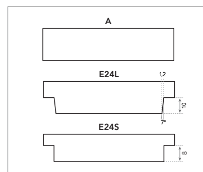
Les bords A et E garantissent un montage rapide et un démontabilité total.
